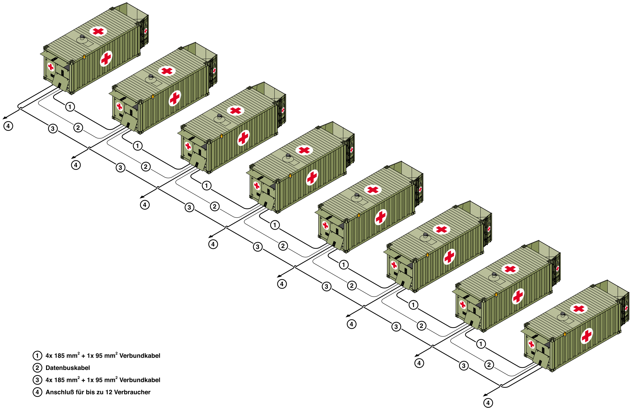
Modulare Sanitätseinrichtung (MSE)
